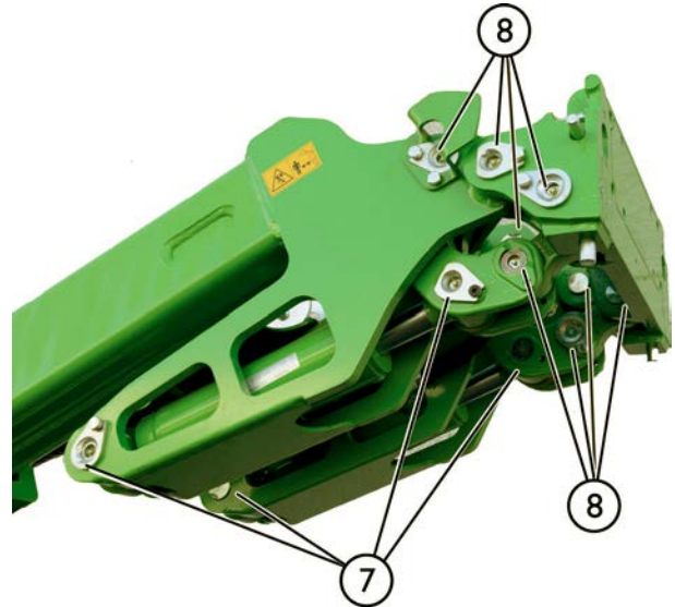
D. Platine d'accrochage et vérins d'inclinaison
